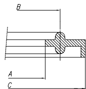
JUNTA RACORD CLAMP CON LAVIO UNION CLAMP SEAL WITH LIP JOINT RACCORD CLAMP AVEC LÈVRE
