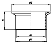
CASQUILLO CLAMP SOLDAR WELDING CLAMP FERRULE CLAMP À SOUDER
